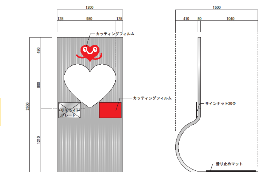
サテライト什器(メイン)レイアウト S=1/20 素材：ステンレスヘアライン(樹脂食仕上げ) マーク：フィルム印刷(樹脂食仕上げ) プレート：発光品取付 ※色コーティング(電着材取付)色確認
